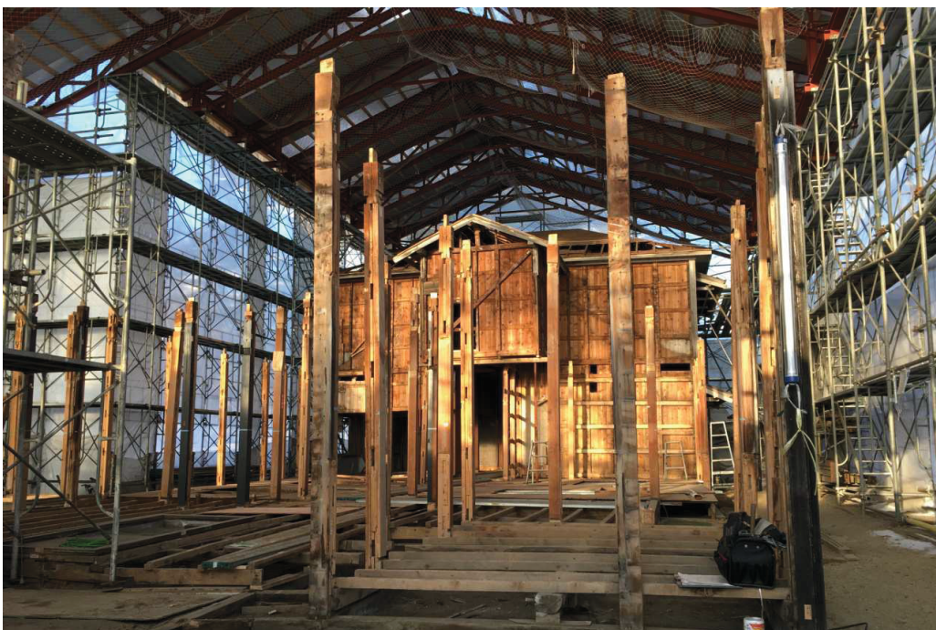
1月25日撮影 工事現場外観(素屋根)
